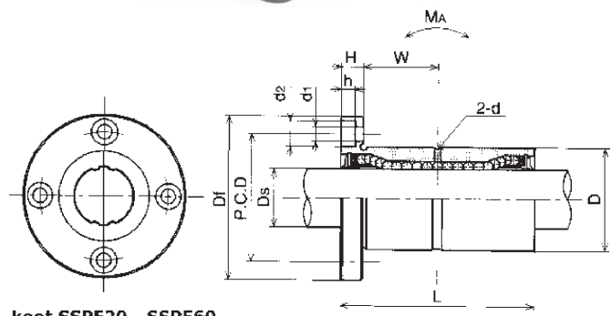
koot SSPF20 - SSPF60
